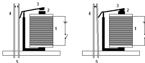
Figura 7: Relé Eletromecânico.
